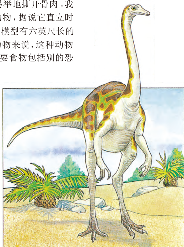
鸵龙
