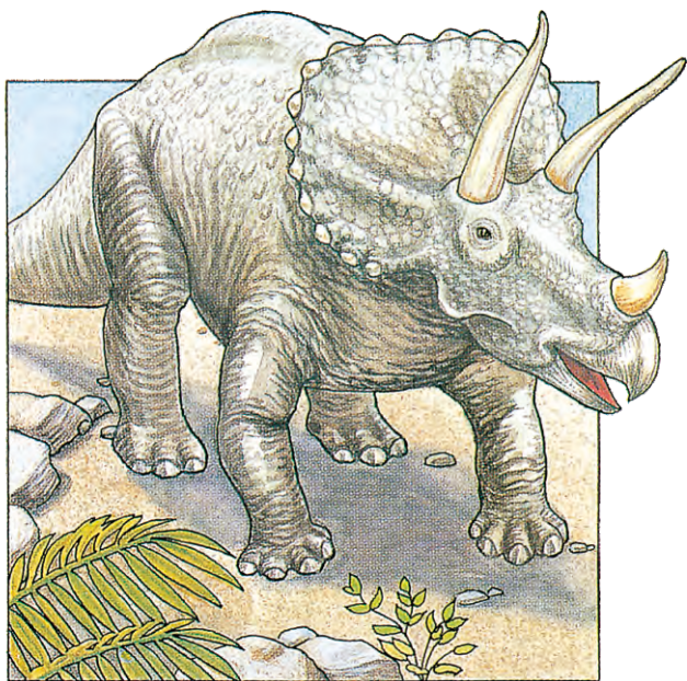
三犄龙
