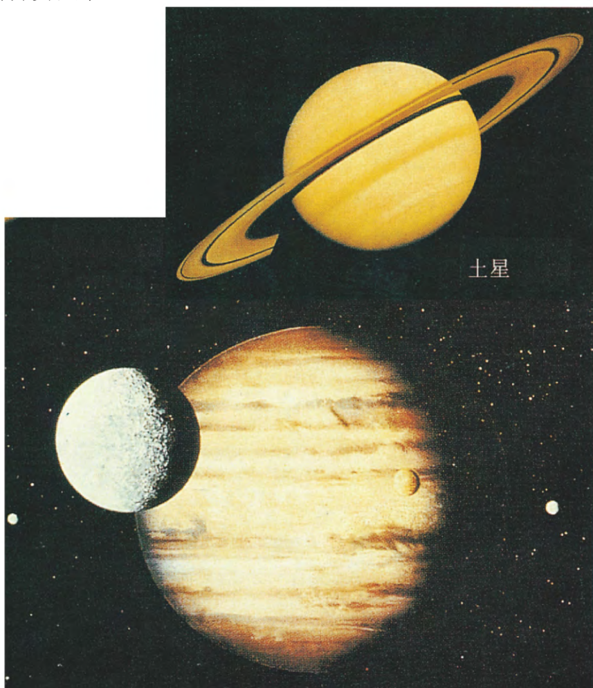
木星和卫星
