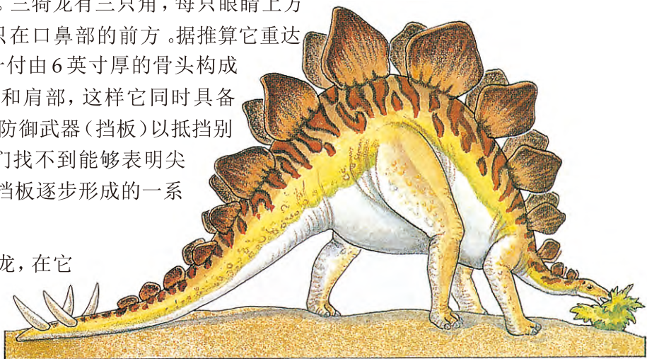
剑龙
