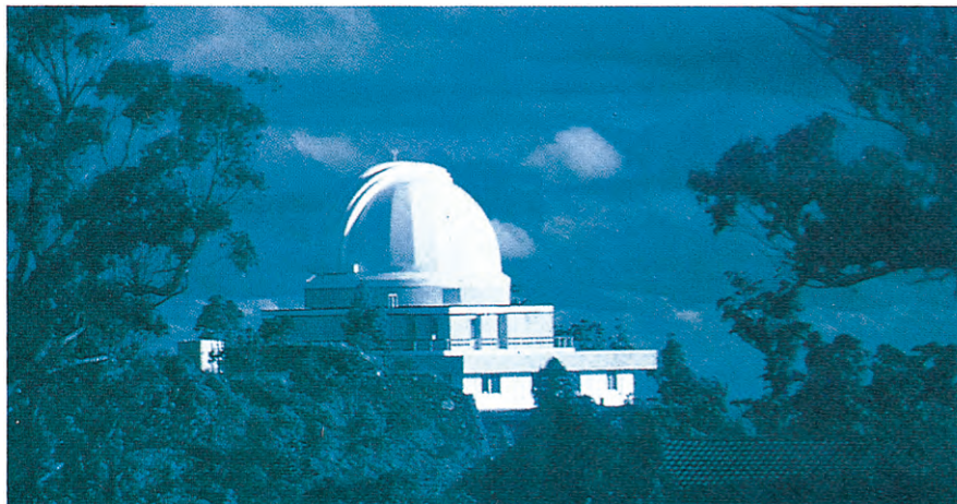
天文台
