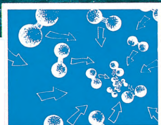
万有引力
