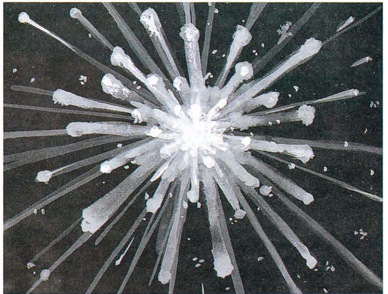
大爆炸理论
